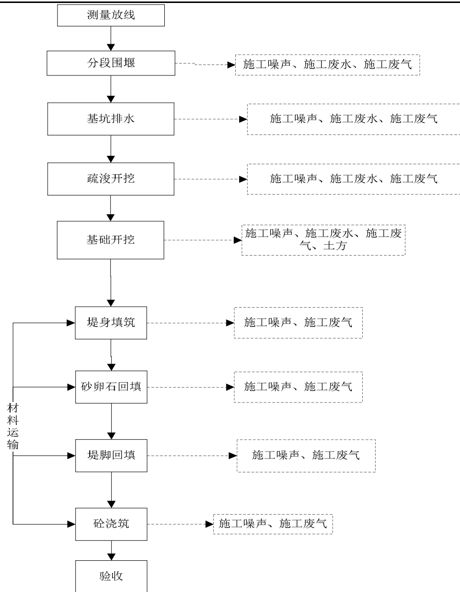
图 2-3 施工流程图
