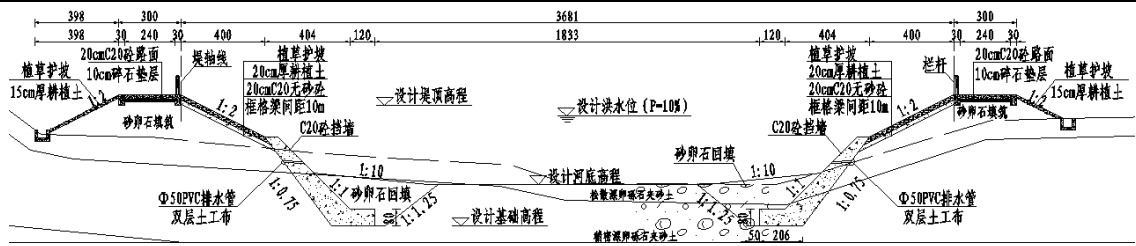
图 2-2 仰斜式挡墙+无砂砼护坡堤型
