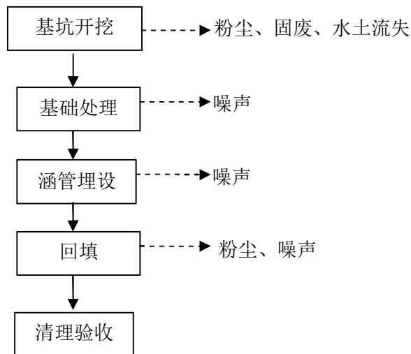
图 2-2 穿堤涵管施工工艺流程及产污位置图
