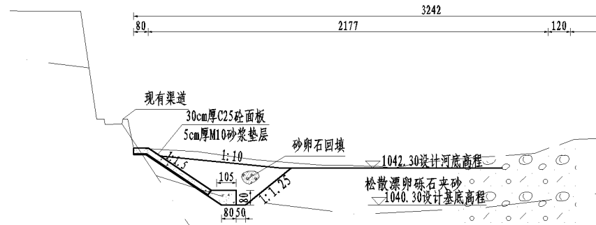
图 2-3 仰斜式挡墙+无砂砼护坡堤型
