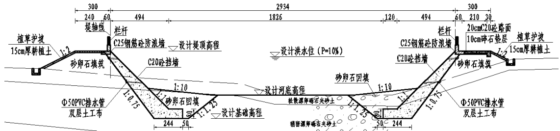
图 2-1 仰斜式挡墙堤型
